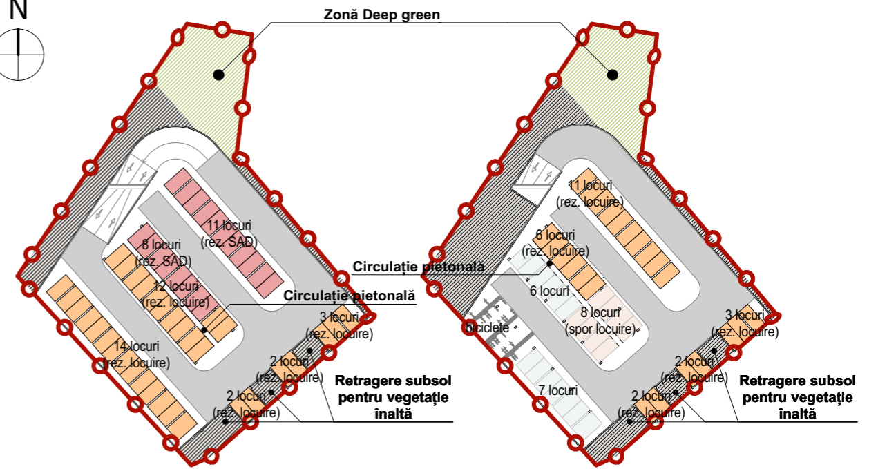
Subsol nivel 1
