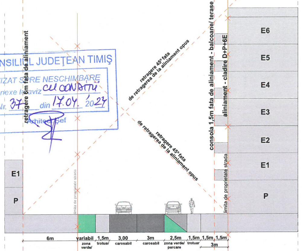
PROFIL STRALAL PROPUȘ STR. LEGUMICULTURII SECȚIUNEA 1-1
