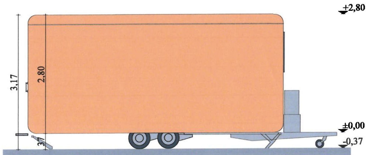
FAȚADĂ POSTERIOARĂ PROPUȘĂ DETALIU REZEMARE PE PLACA DE BETON CONSTRUCȚIE PROVIZORIE PE ROȚI (TIP RULOTĂ)
