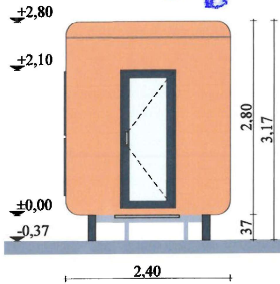
FAȚADĂ LATERALĂ DREAPTA PROPUȘĂ
