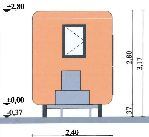
FAȚADĂ LATERALĂ STÂNGA PROPUȘĂ
