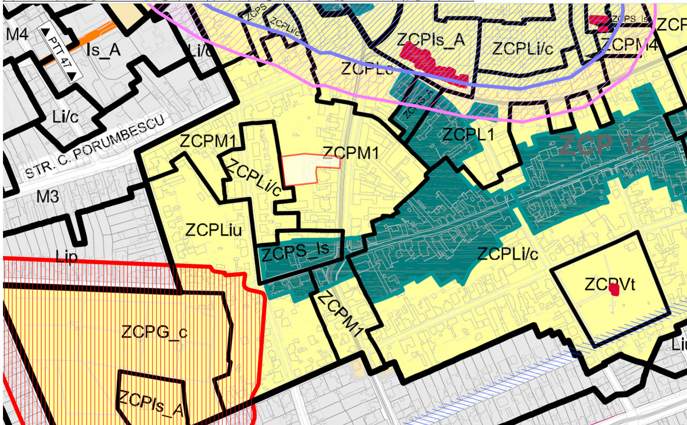
Incadrare in PUG nou Mun. Timisoara Zona ZCP M1 - Iosefin/Fabrik/Zona constructibila protejata, Zona mixta cu regim de construire inchis adiacenta principalelor artere de trafic
