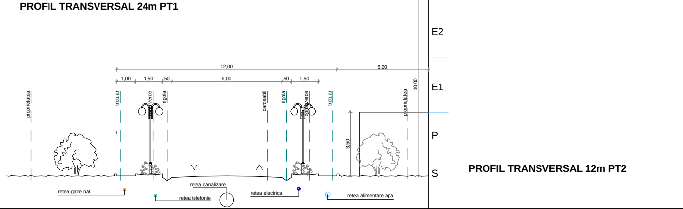
PROFIL TRANSVERSAL 24m PT1
