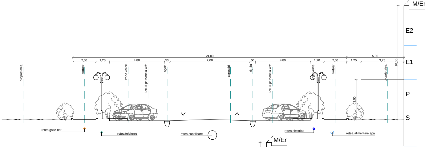
PROFIL TRANSVERSAL 24m PT1
