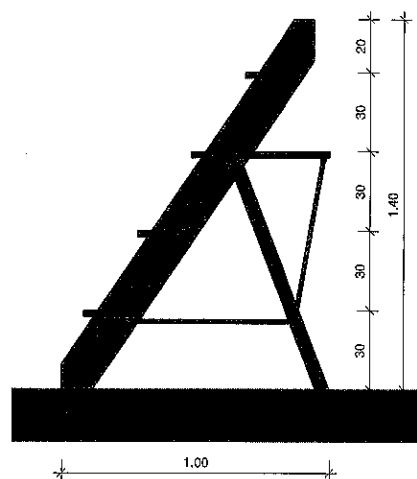
Secțiune transversală
