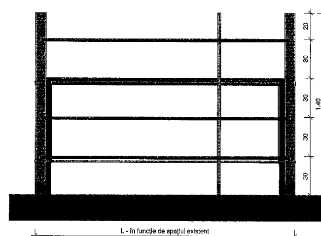
Vedere frontală
