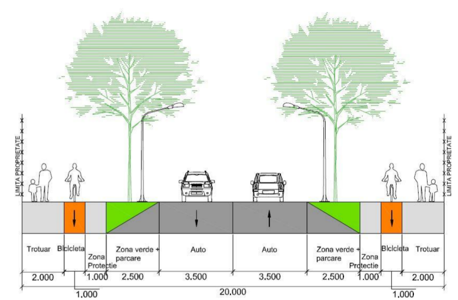
Profil stradal propus pentru drumul cedat
