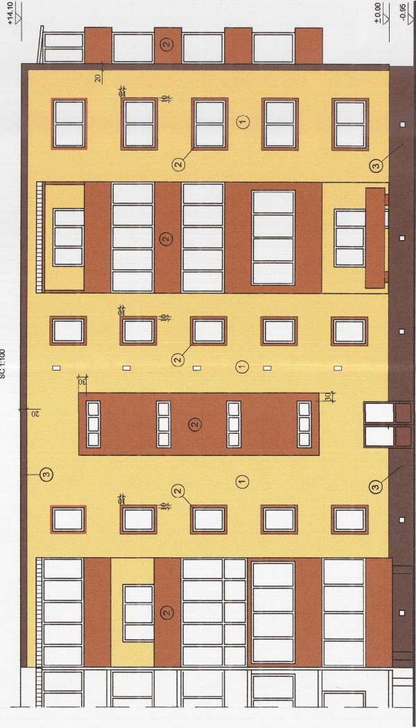
FATADA POSTERIOARA - Propunere SC 1:100
