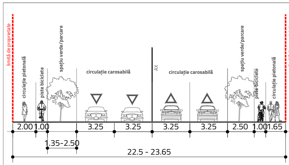
Profil E-E' REORGANIZARE PROPUȘĂ - Str. Popa Șapcă
