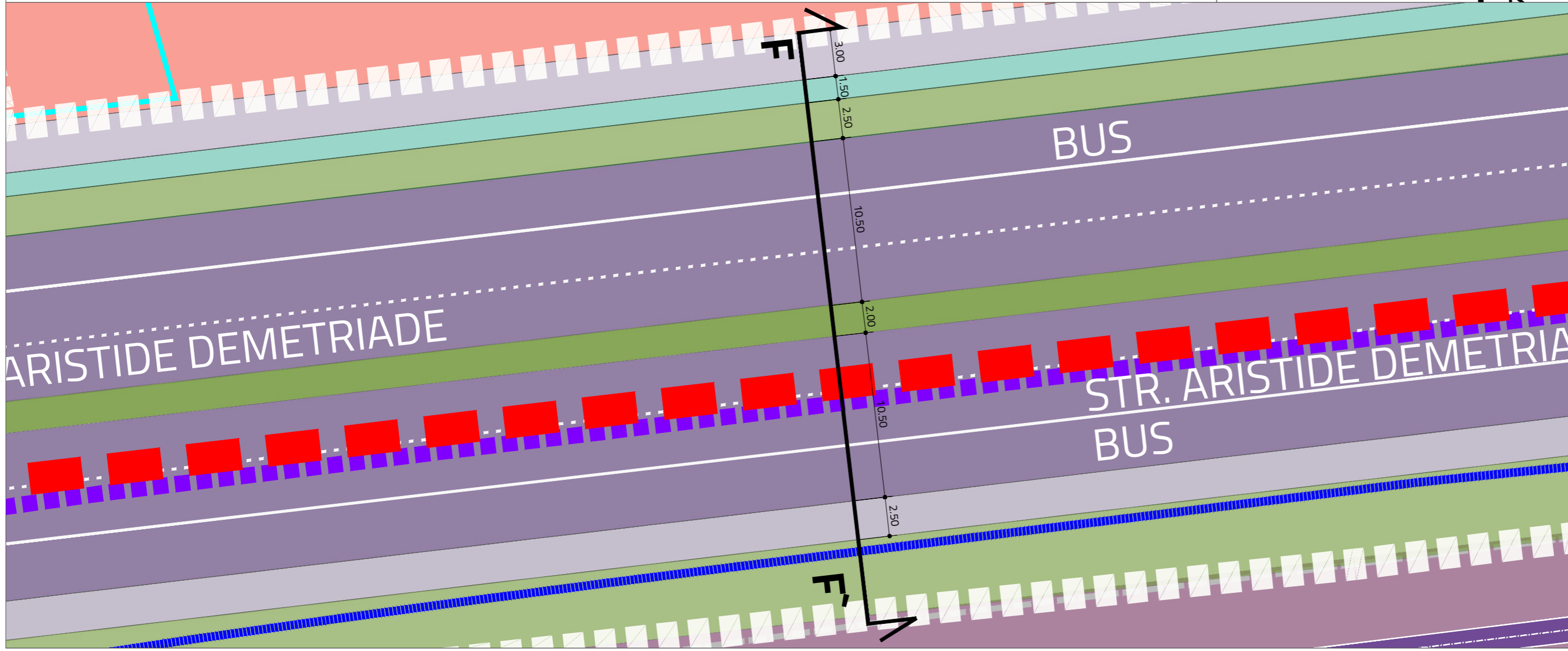
Profil F-F' REORGANIZARE PROPUȘĂ - Str. Aristide Demetriade
