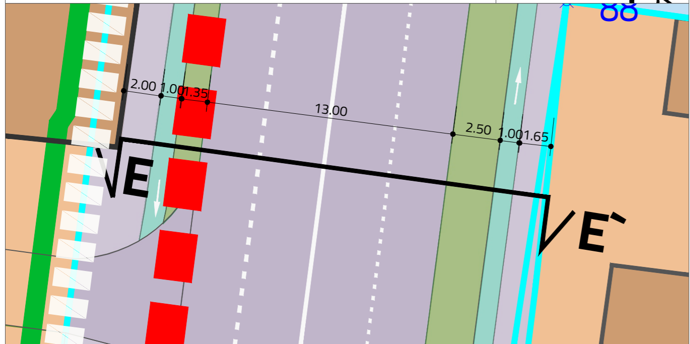
Profil E-E' REORGANIZARE PROPUȘĂ - Str. Popa Șapcă
