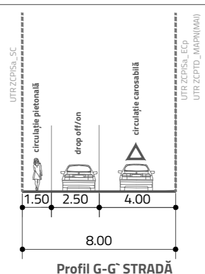
Profil G-G' STRADĂ DROP ON/OFF - DO. 1
