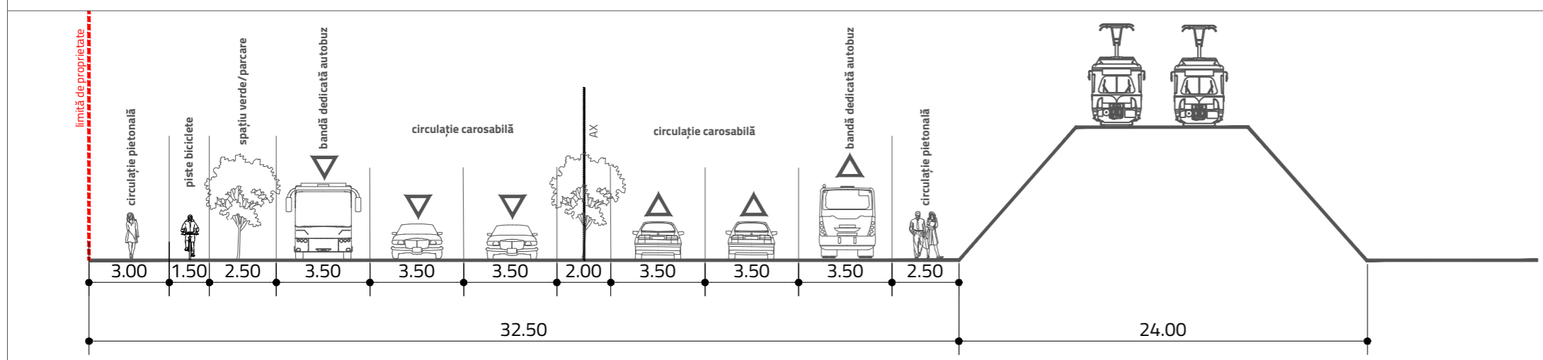
Profil F-F' REORGANIZARE PROPUȘĂ - Str. Aristide Demetriade
