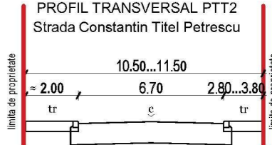
Profiluri transversale de drum existente
