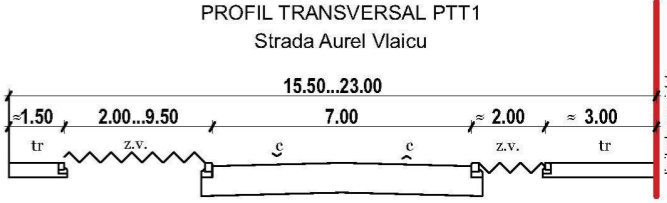
Profiluri transversale de drum existente
