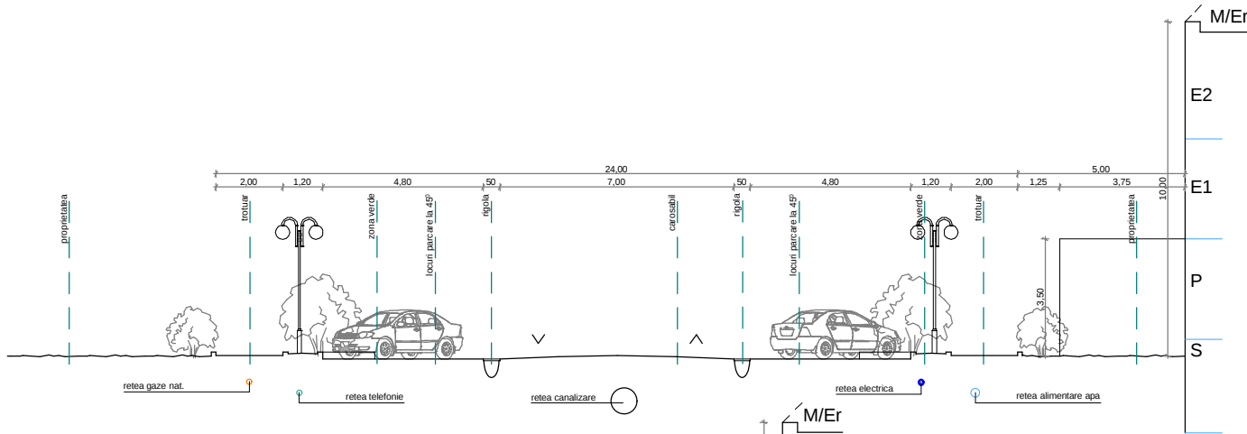
PROFIL TRANSVERSAL 24m PT1
